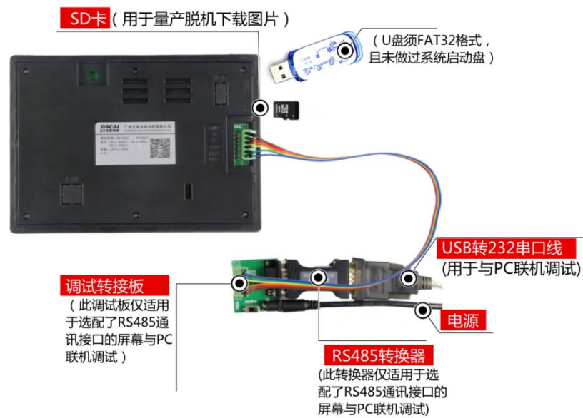
图 1-4 RS485 调试工具图
