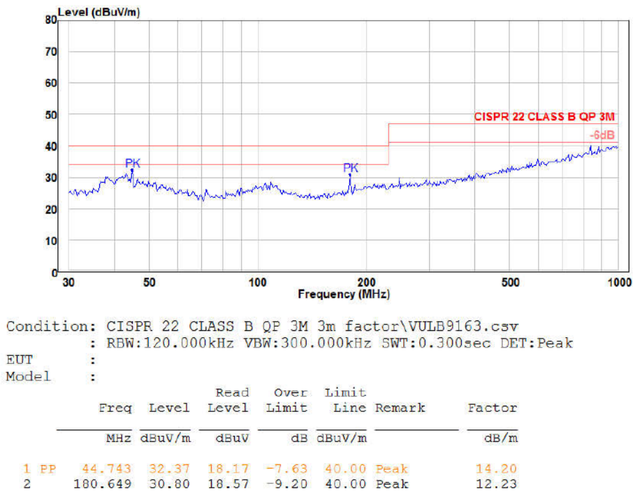
图 6-7 辐射测试垂直方向
