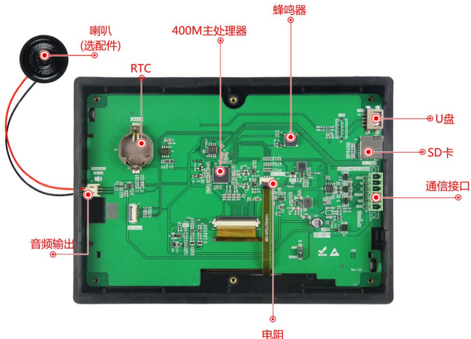
图 1-2 硬件配置图
