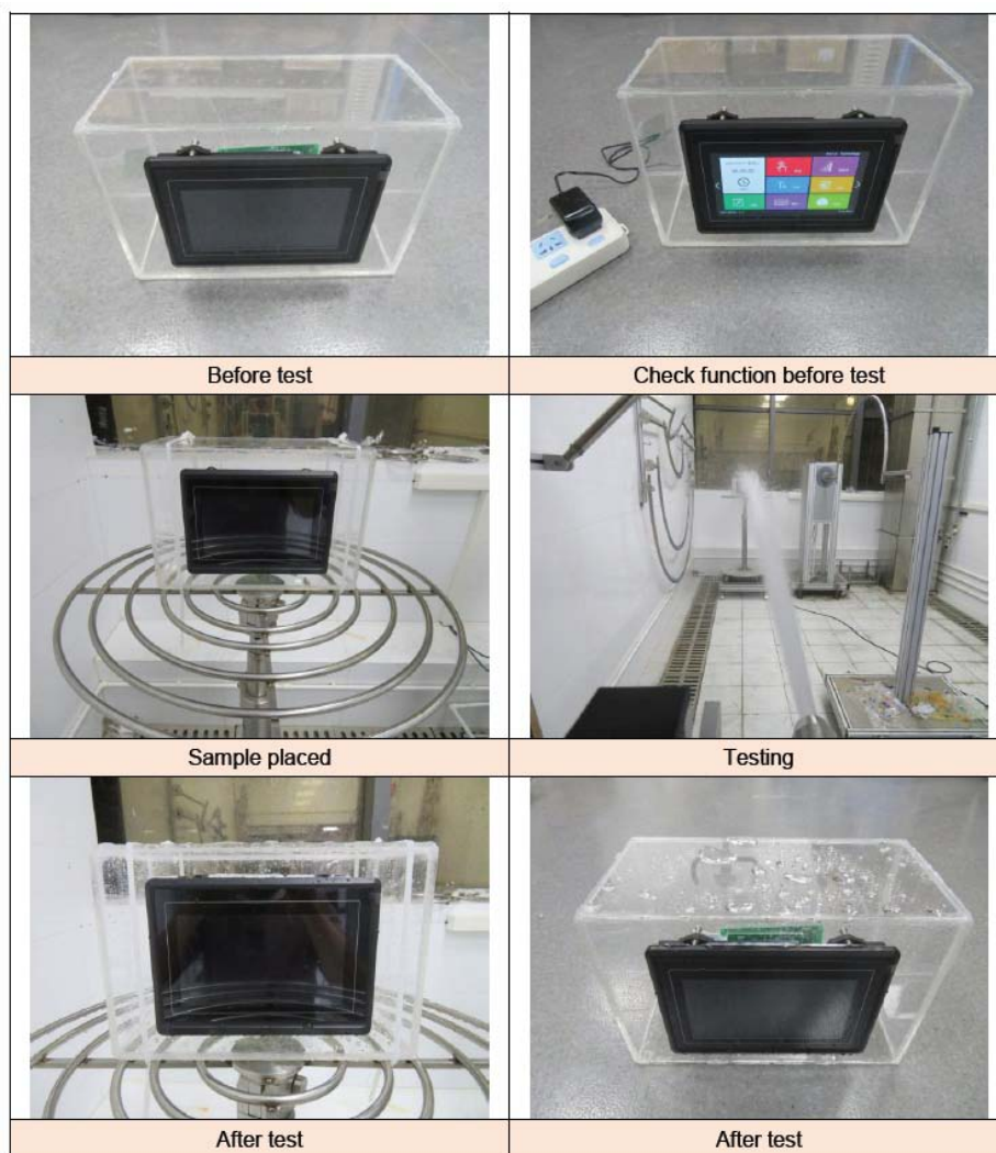
图 6-8 防水测试图
