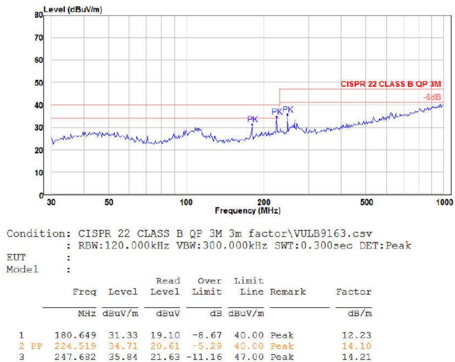
图 6-6 辐射测试水平方向
